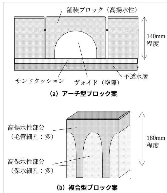
図5 保水と毛管吸水をコントロールする舗装ブロックの形態
